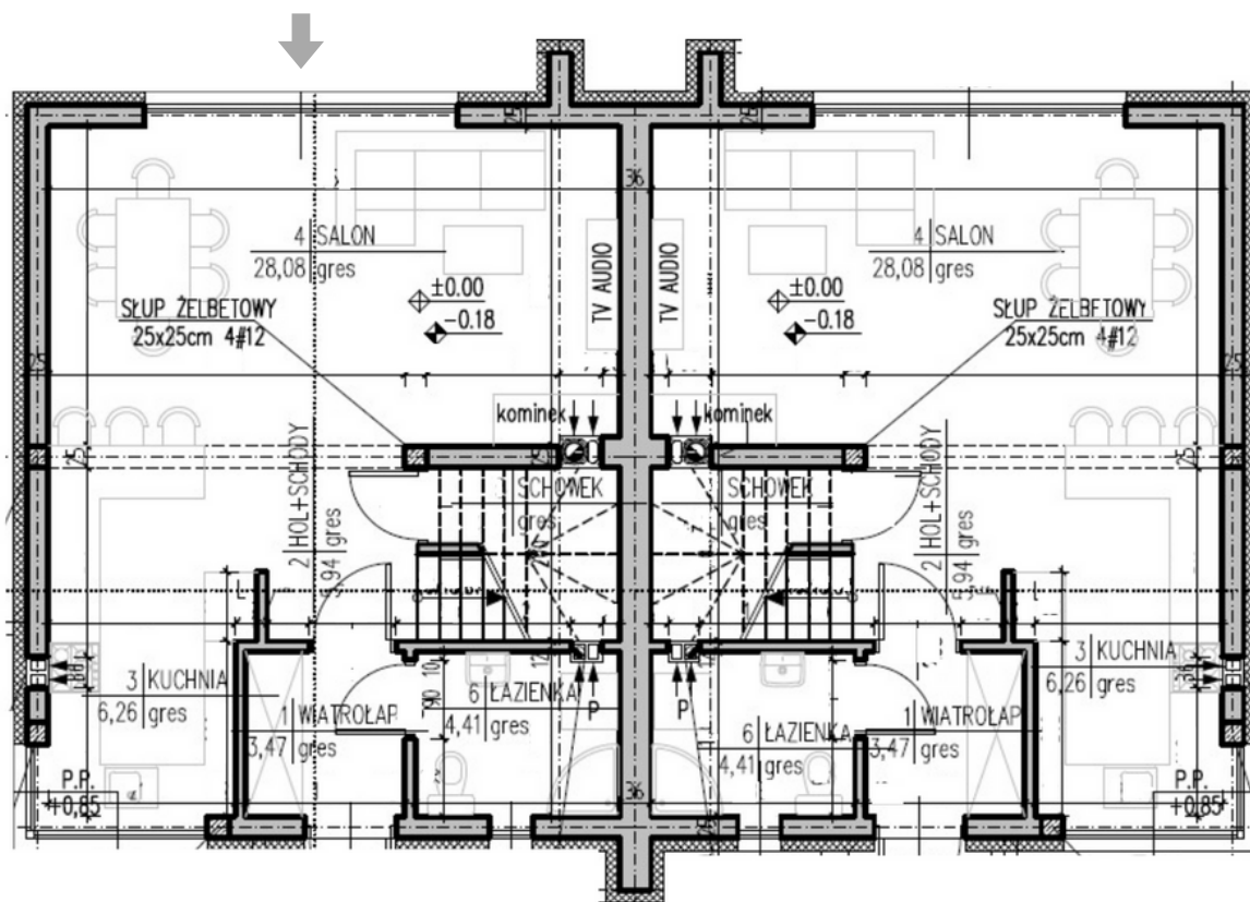
Rzut parter
