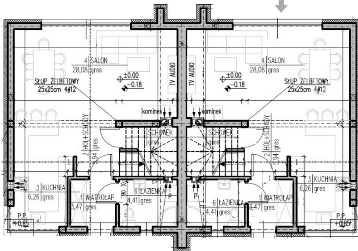
Rzut parter
