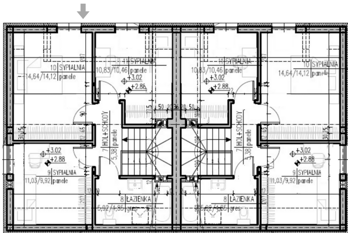
Rzut poddasza
