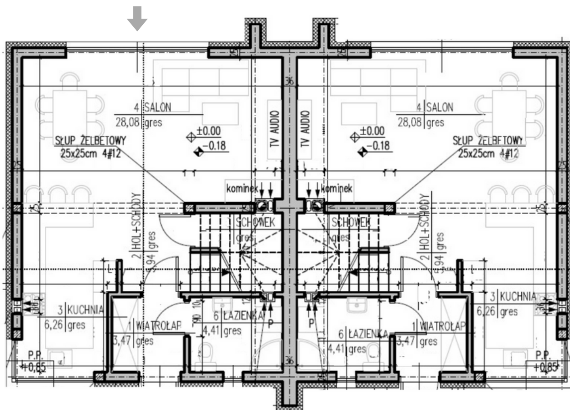
Rzut parter
